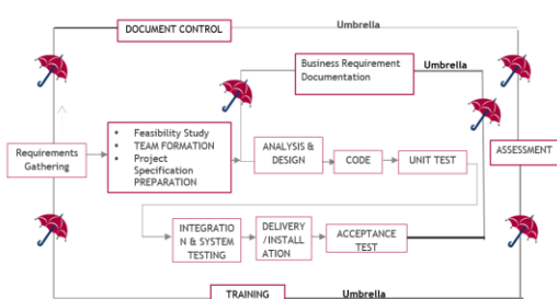
Fig 1: SDLC (Umbrella Model)
